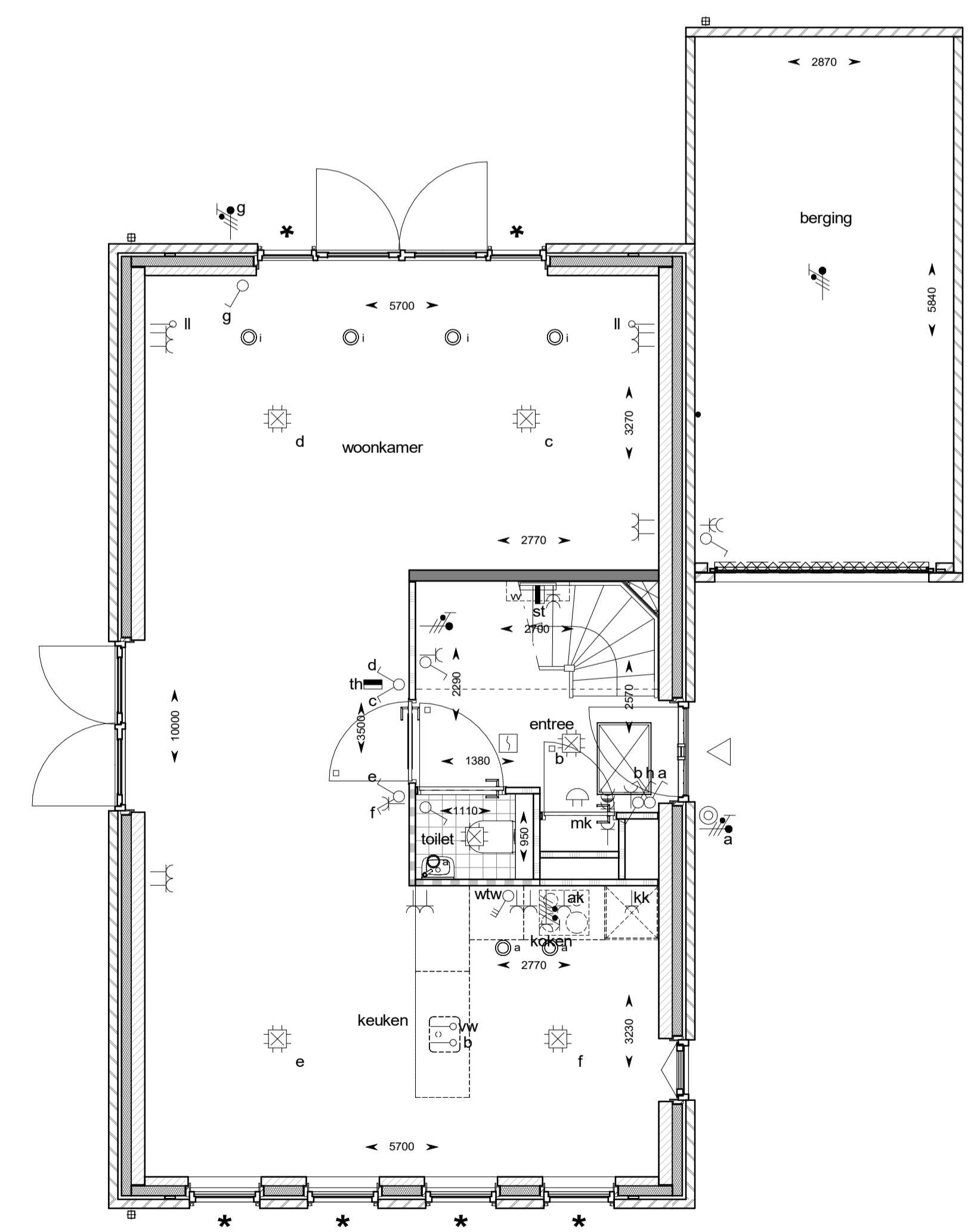
begane grond
