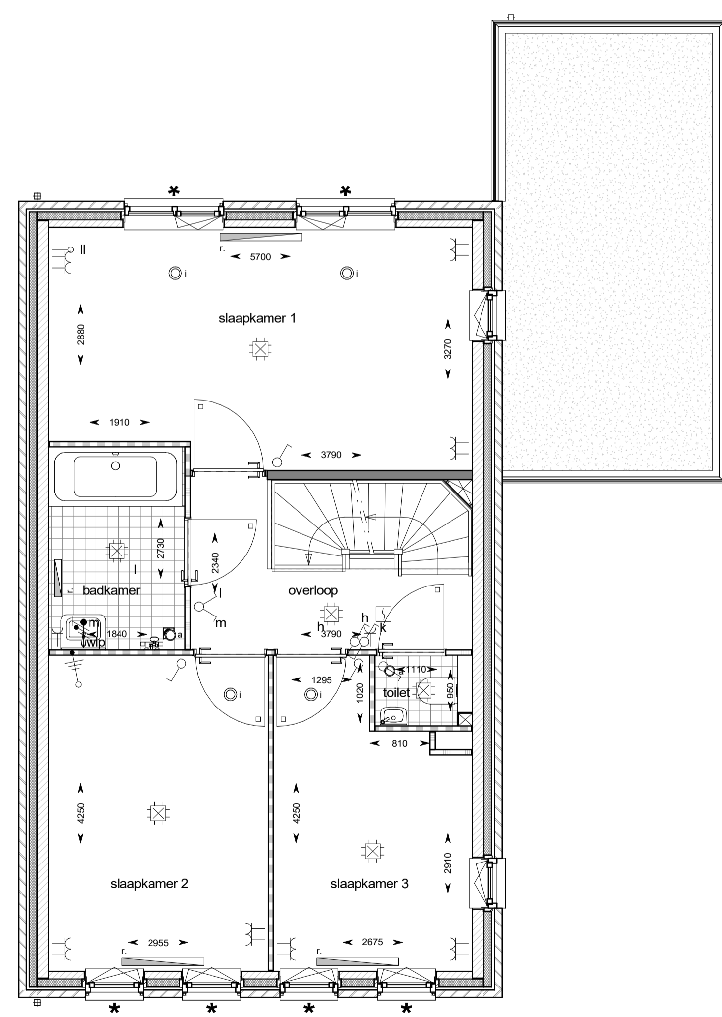
eerste verdieping
