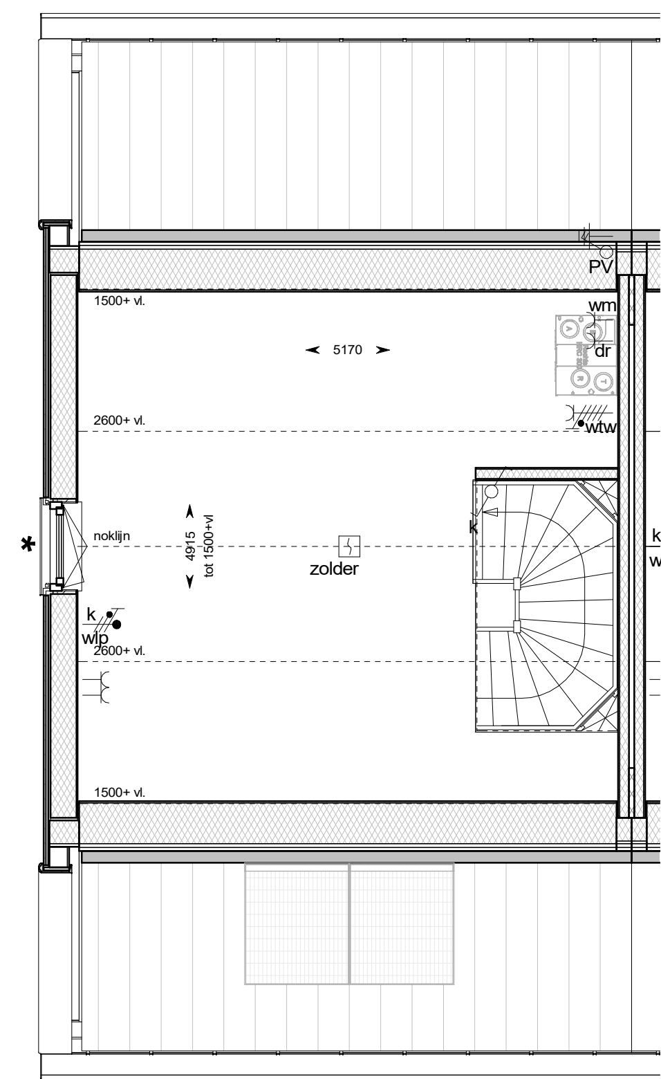
tweede verdieping
