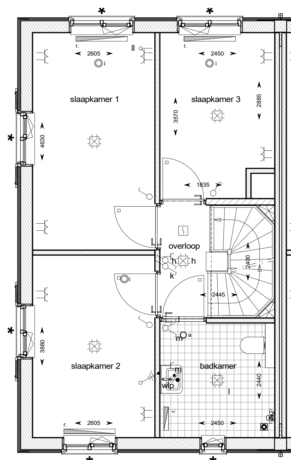
eerste verdieping
