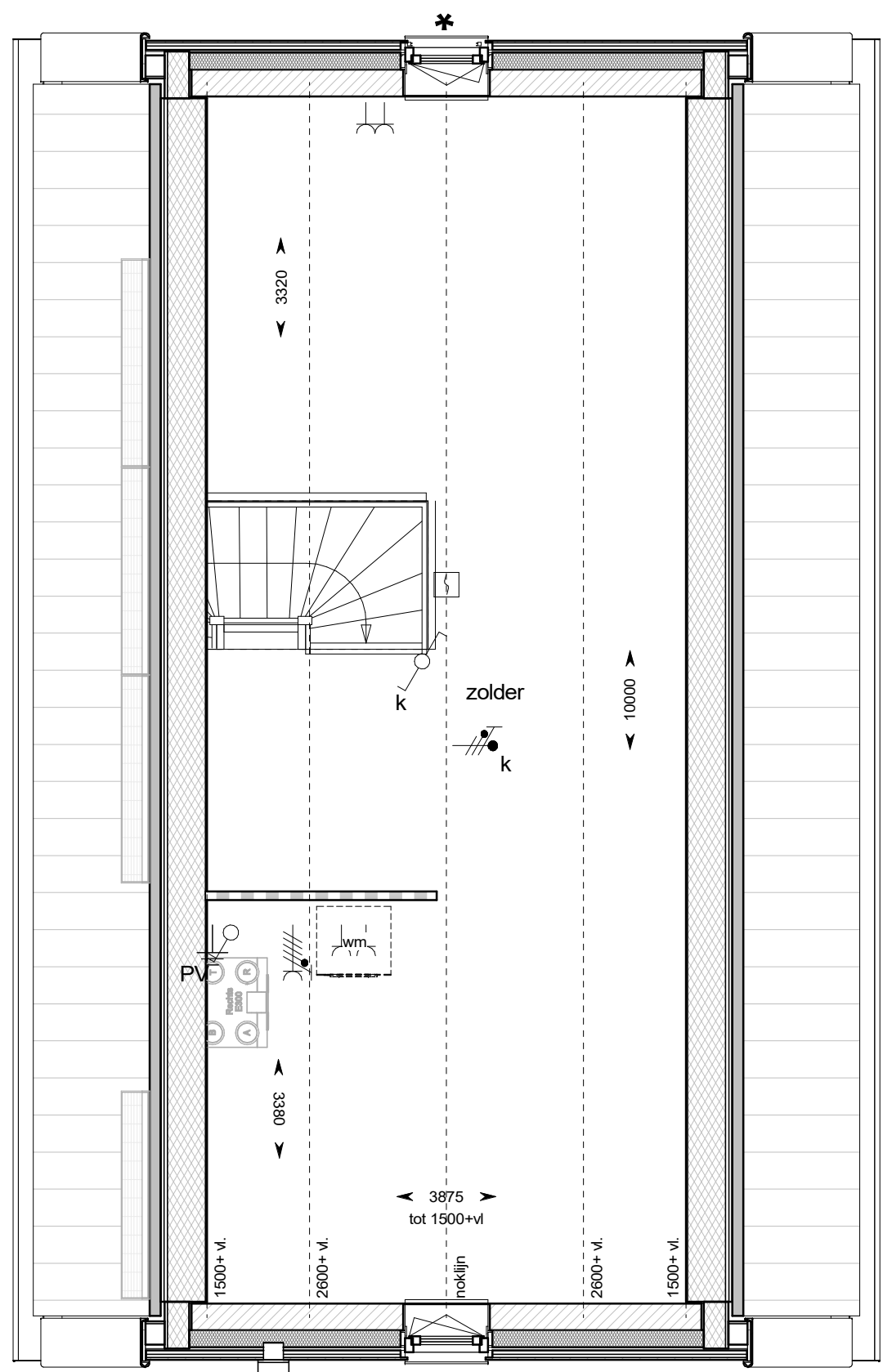
tweede verdieping
