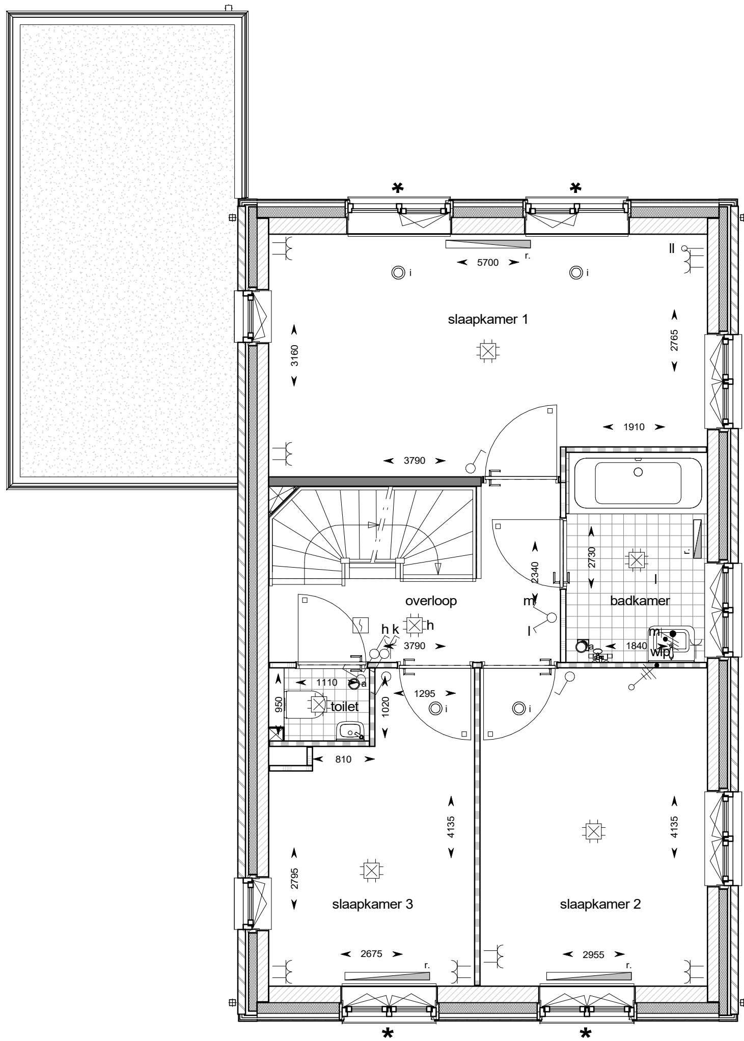
eerste verdieping
