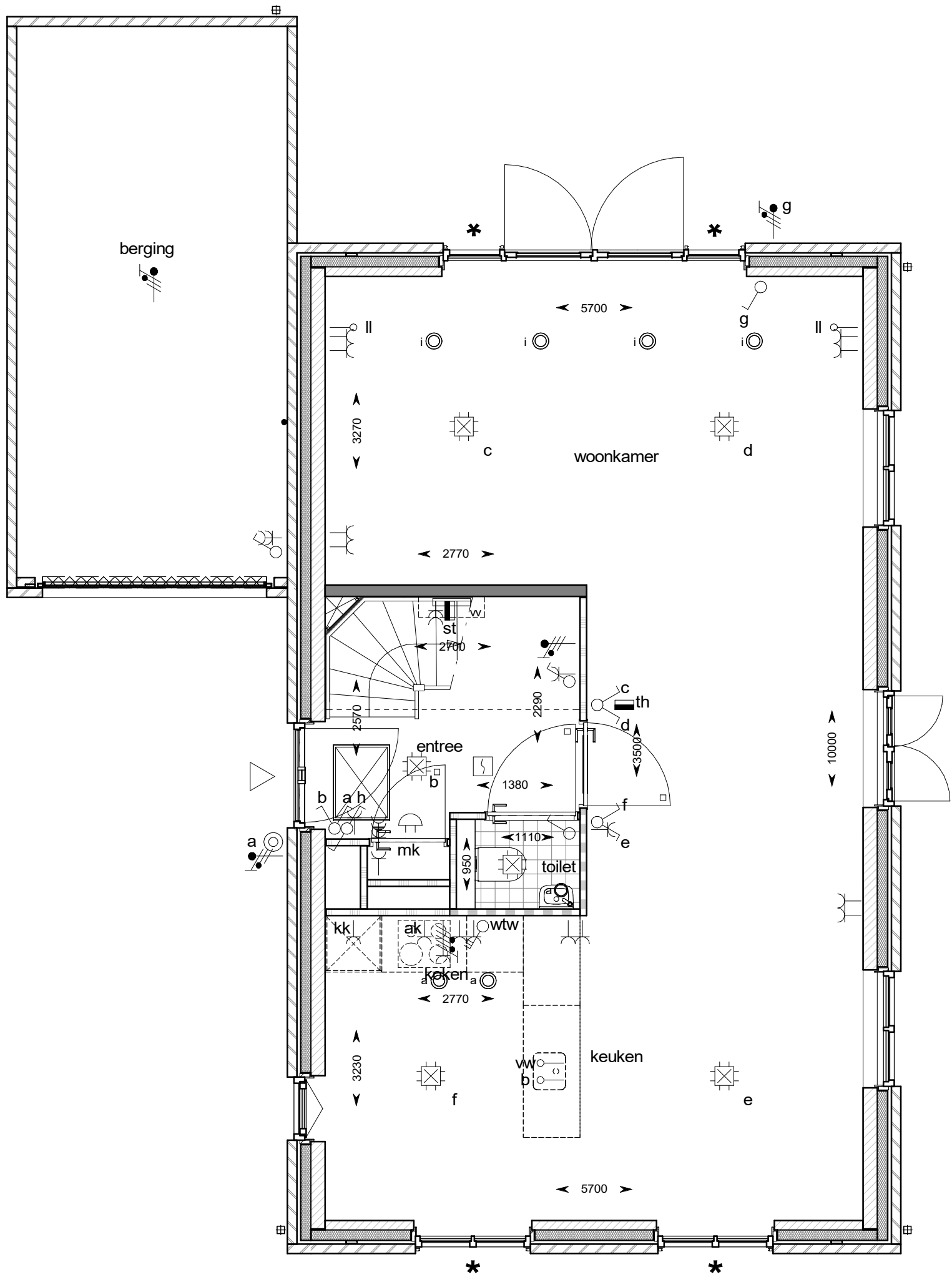
begane grond
