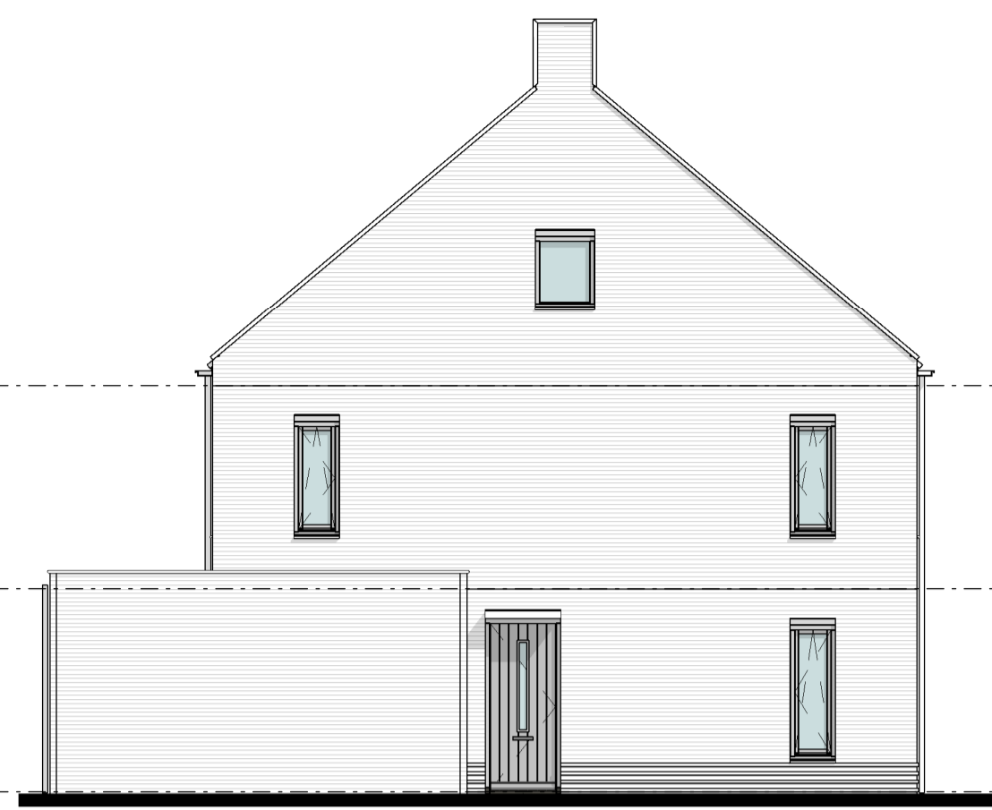
kopgevel
