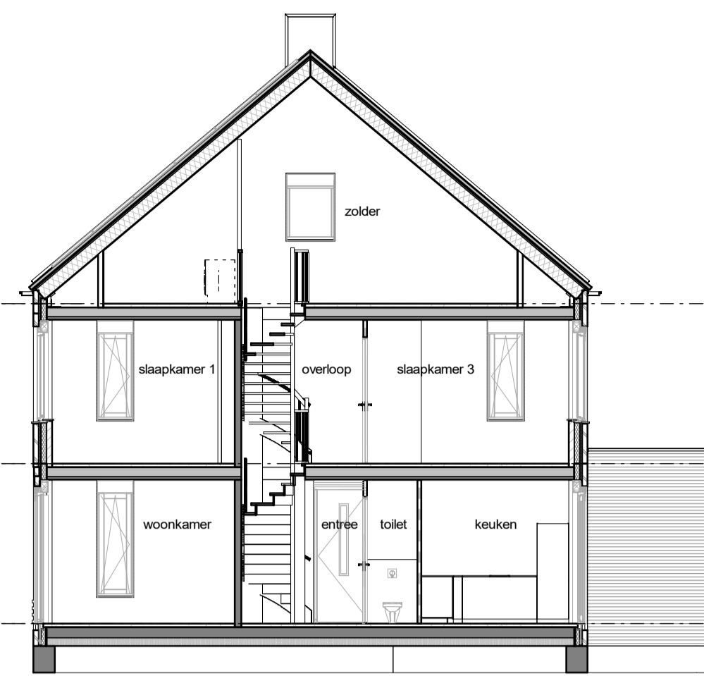
doorsnede
