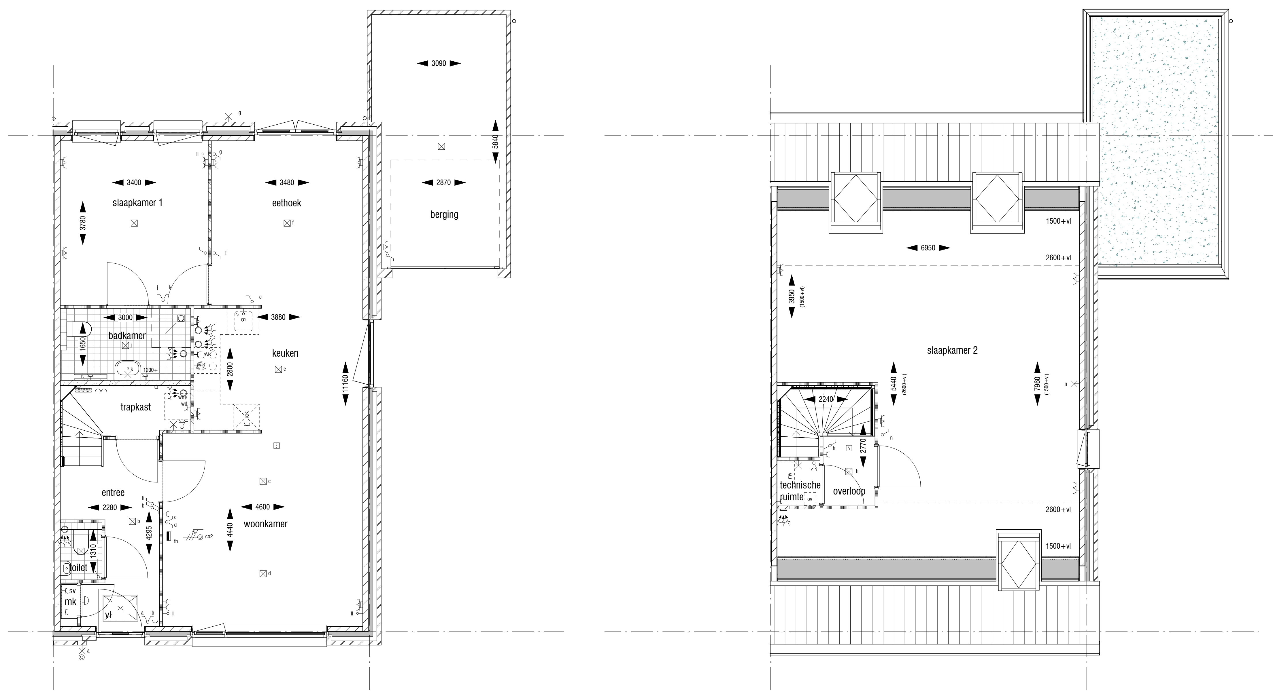
begane grond
