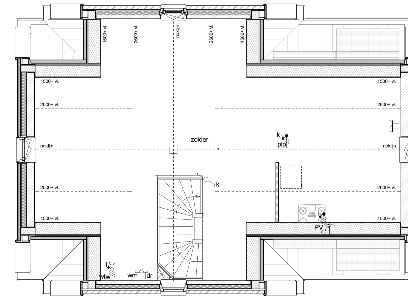
tweede verdieping
