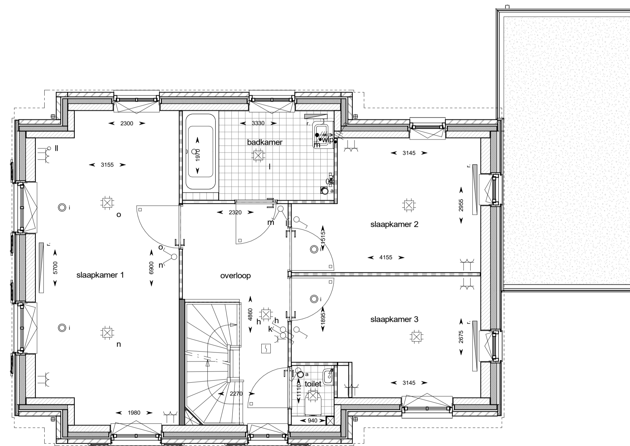
eerste verdieping
