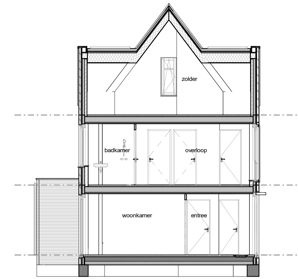
doorsnede
