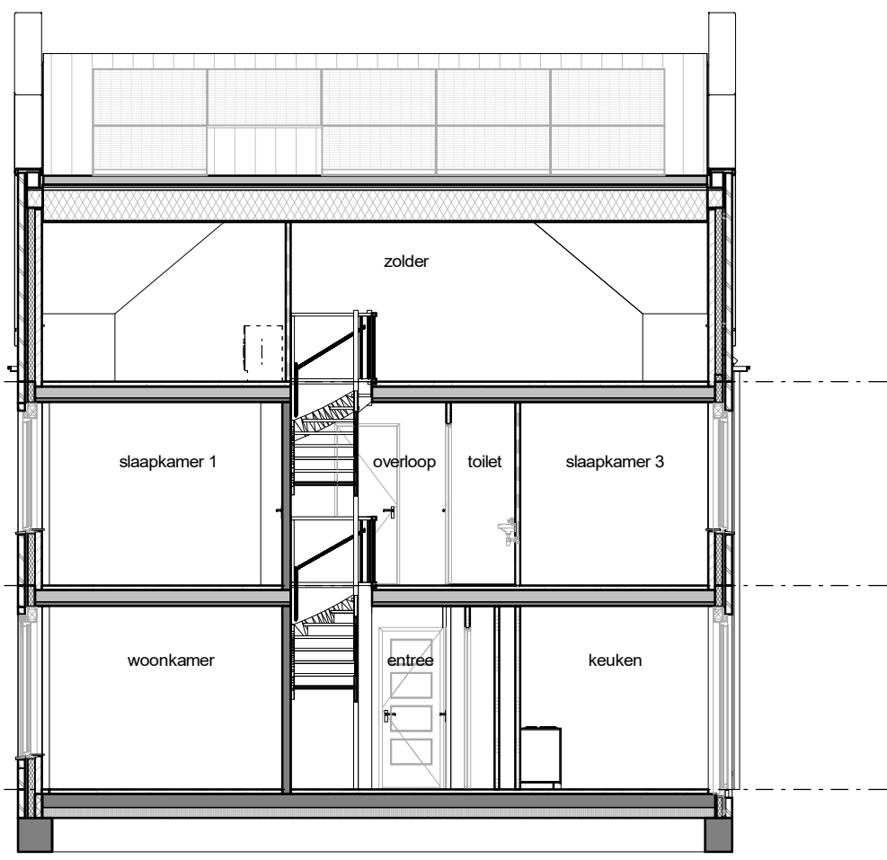
doorsnede
