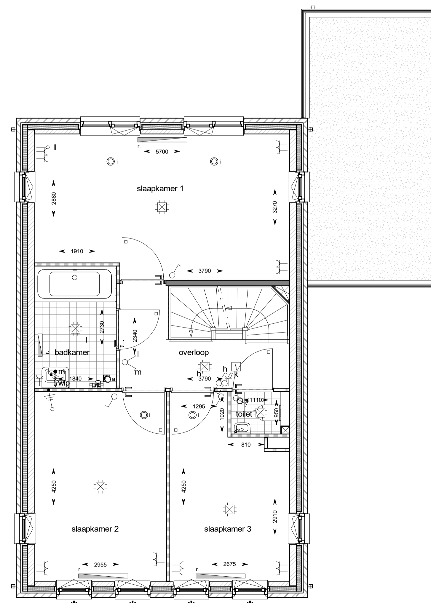
eerste verdieping
