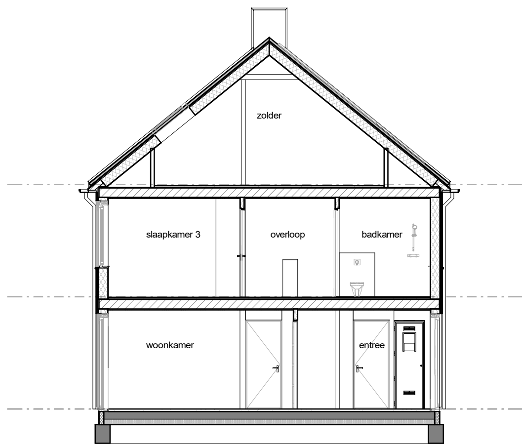
doorsnede
