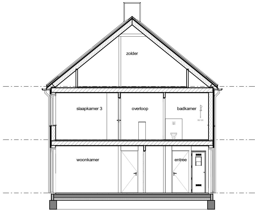
doorsnede
