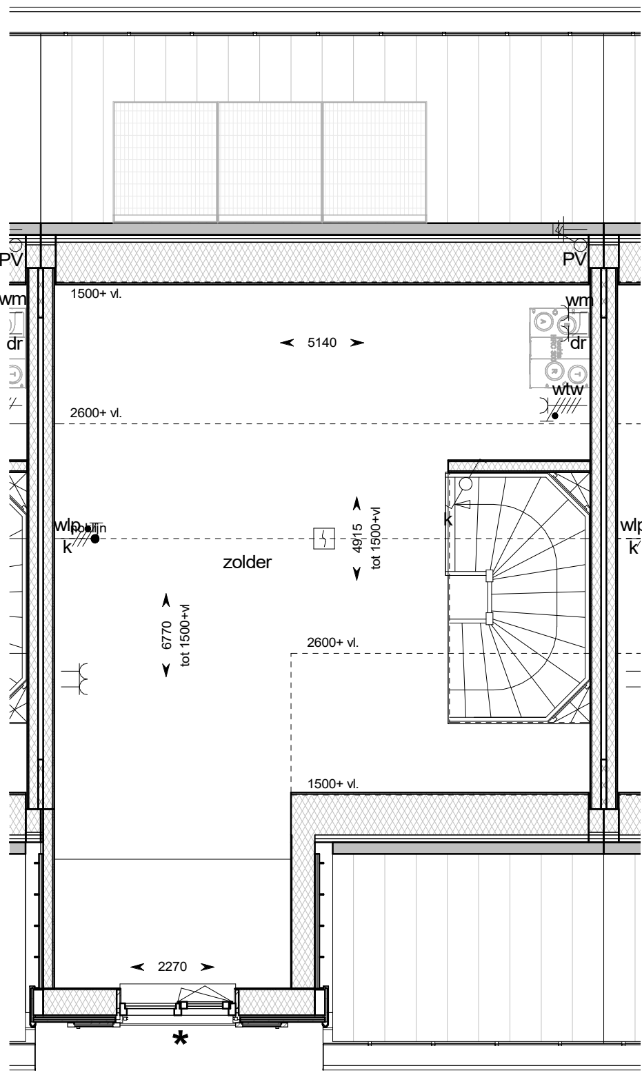
tweede verdieping
