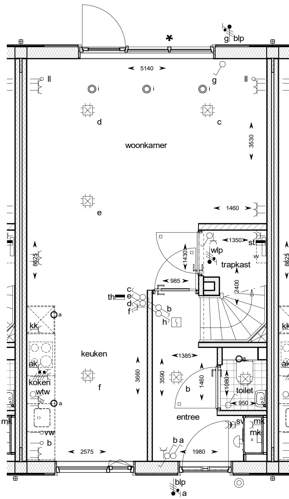
begane grond
