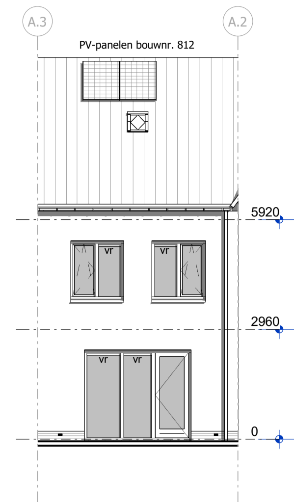
achtergevel
