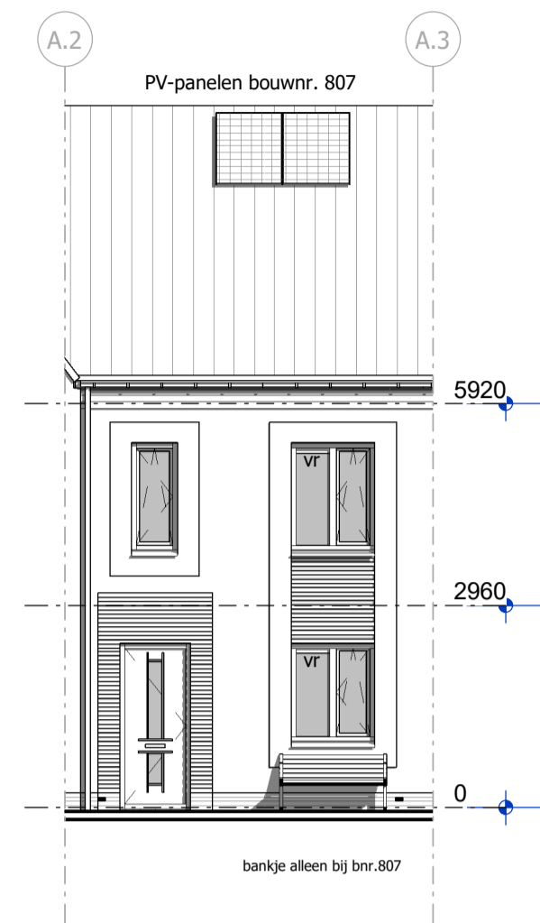
voorgevel
