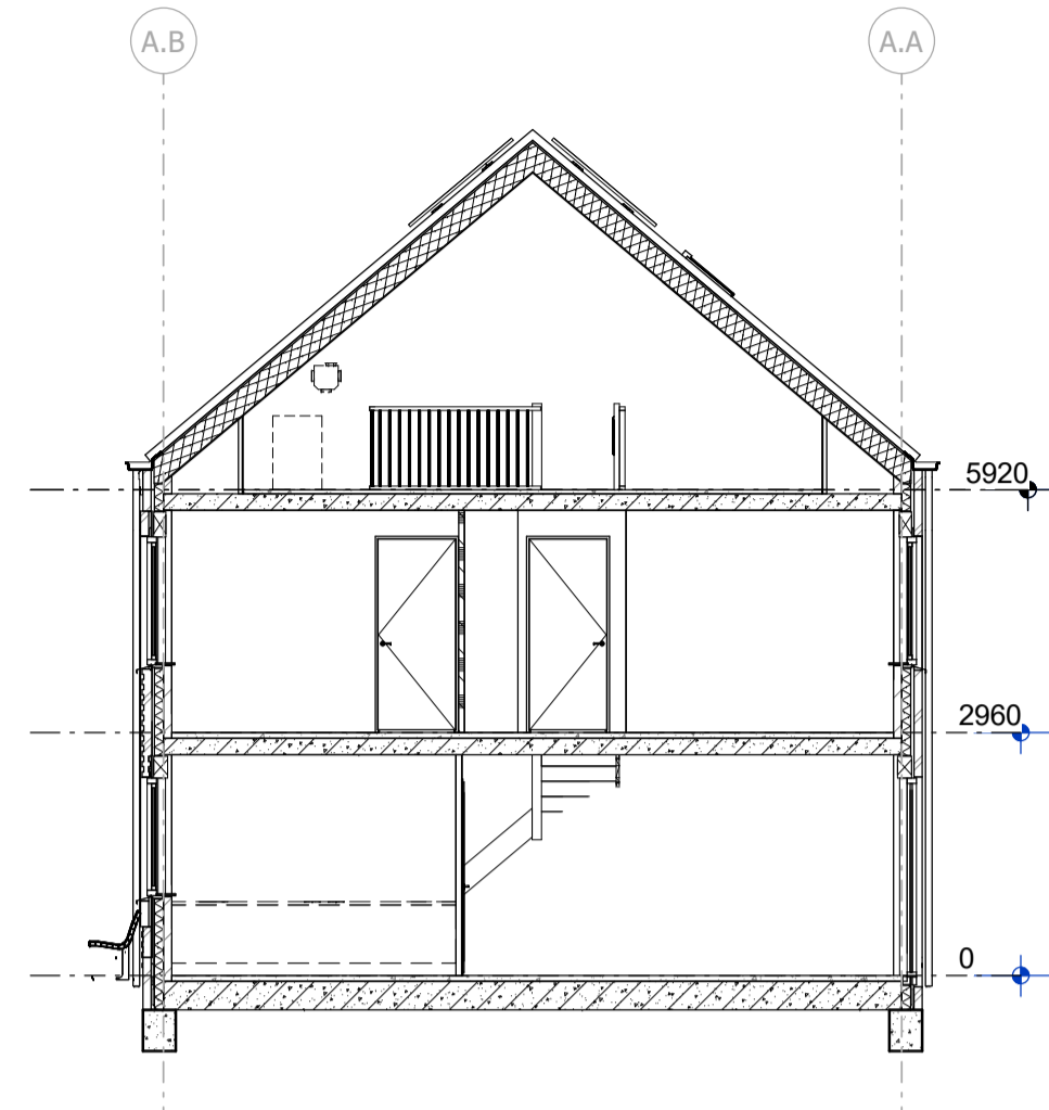
doorsnede A-A
