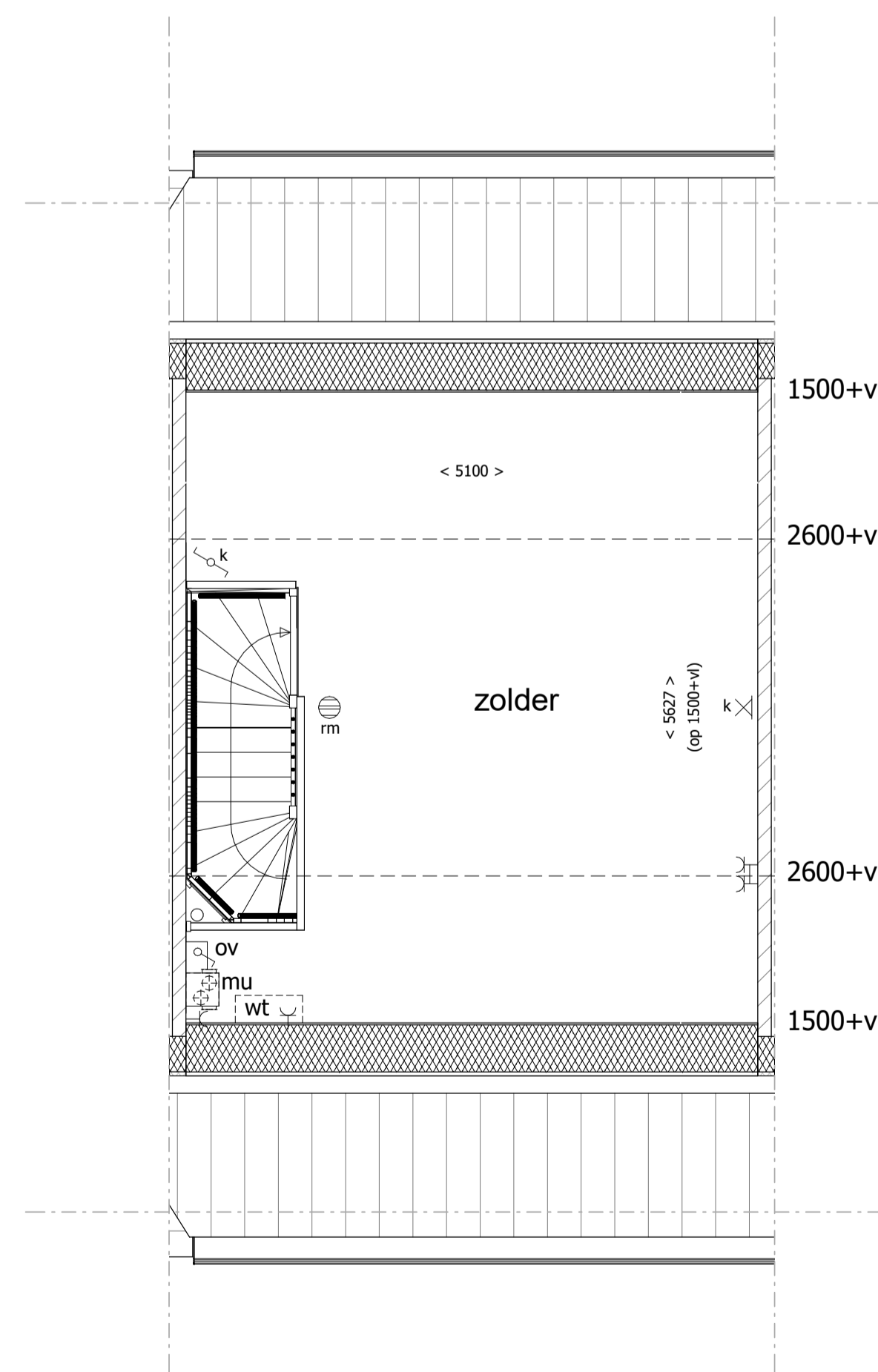
2e verdieping
