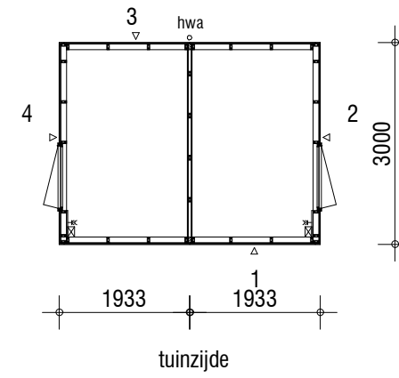
plattegrond dubbele berging
