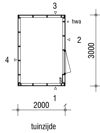
plattegrond berging
