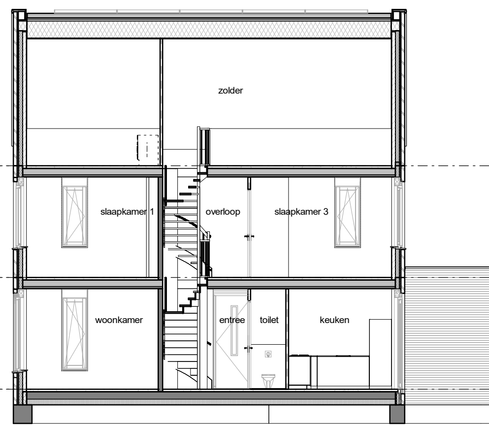
doorsnede
