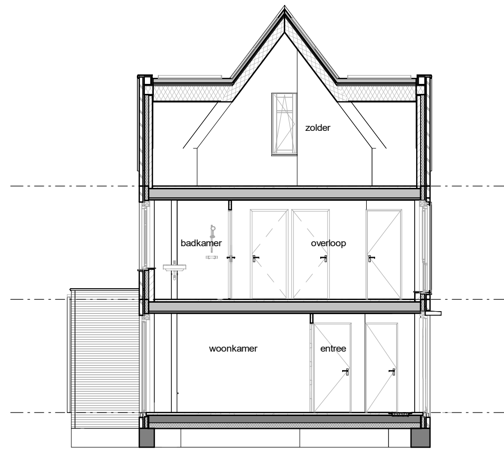
doorsnede
