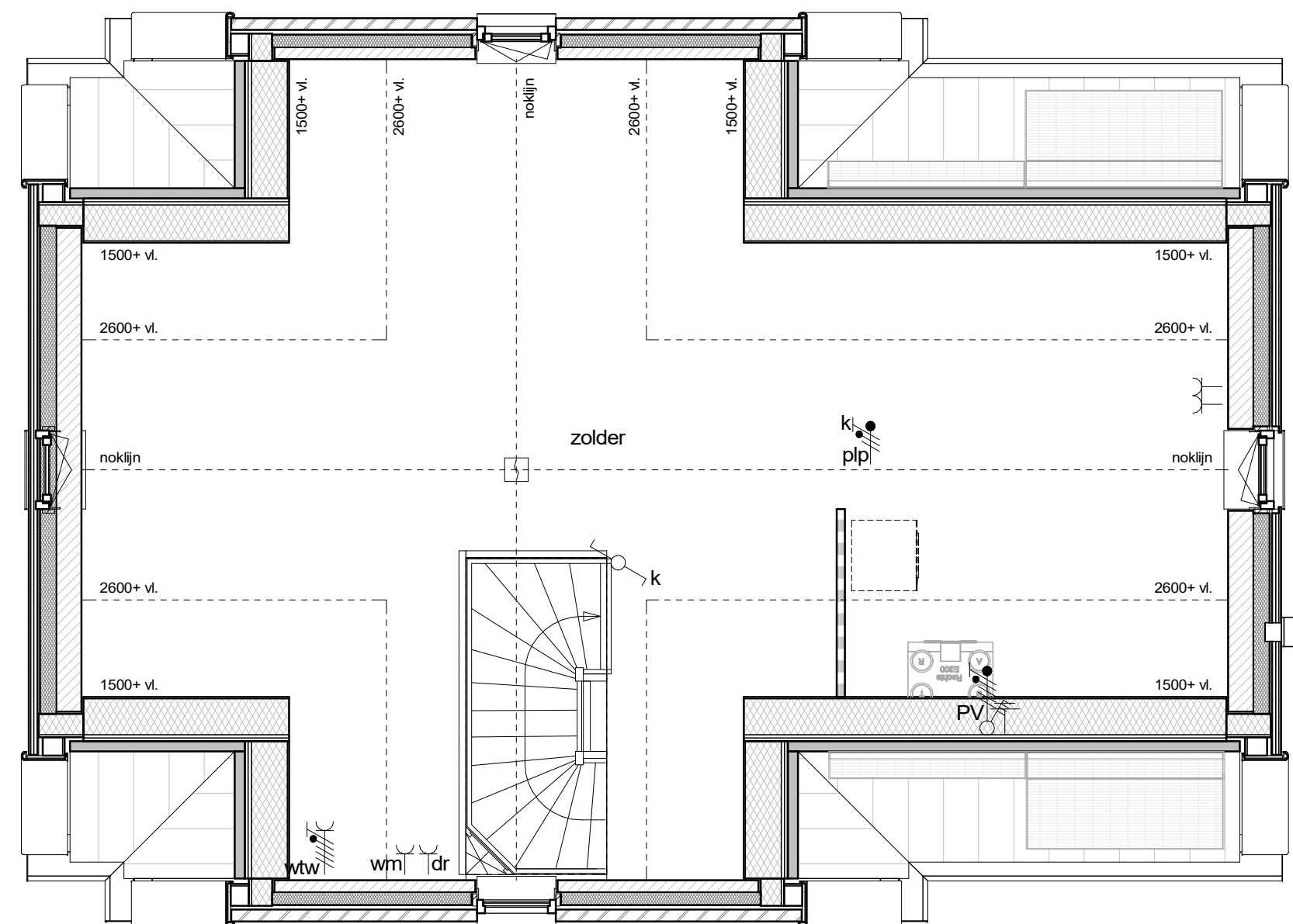
tweede verdieping
