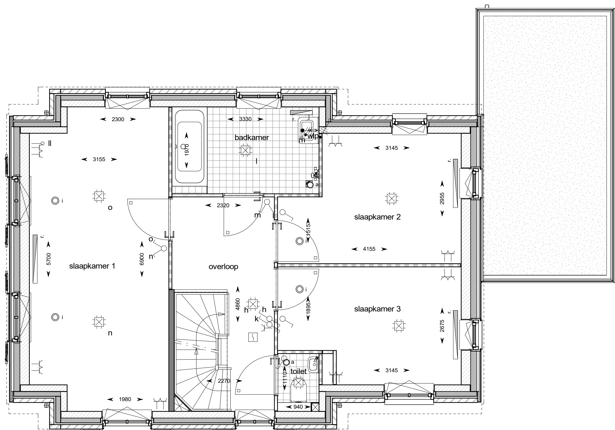
eerste verdieping
