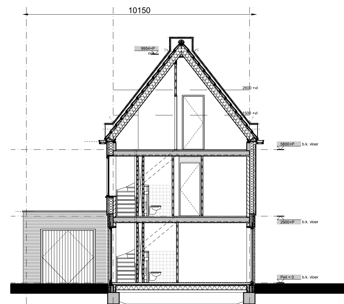
doorsnede A-A
