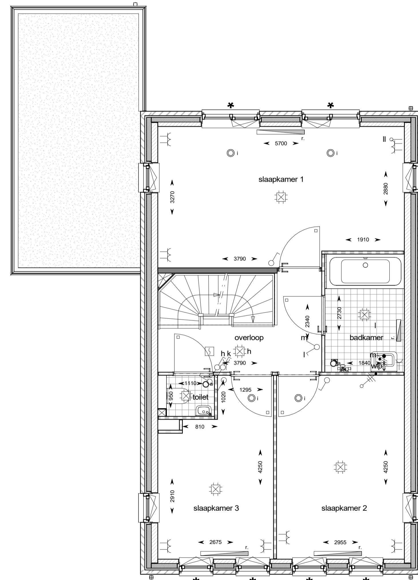
eerste verdieping
