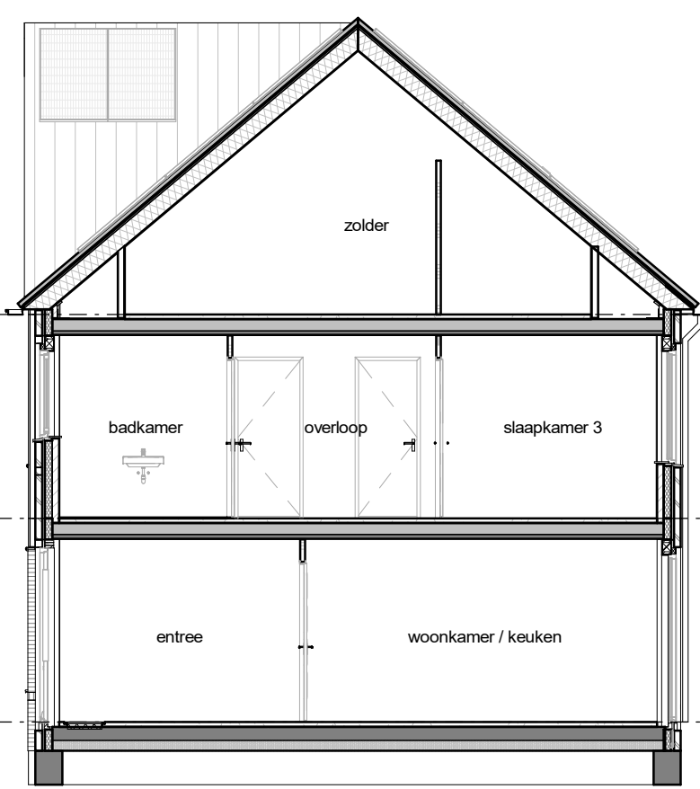
doorsnede
