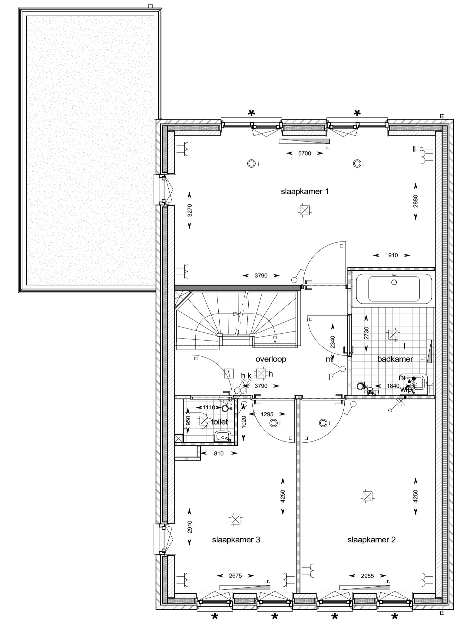
eerste verdieping
