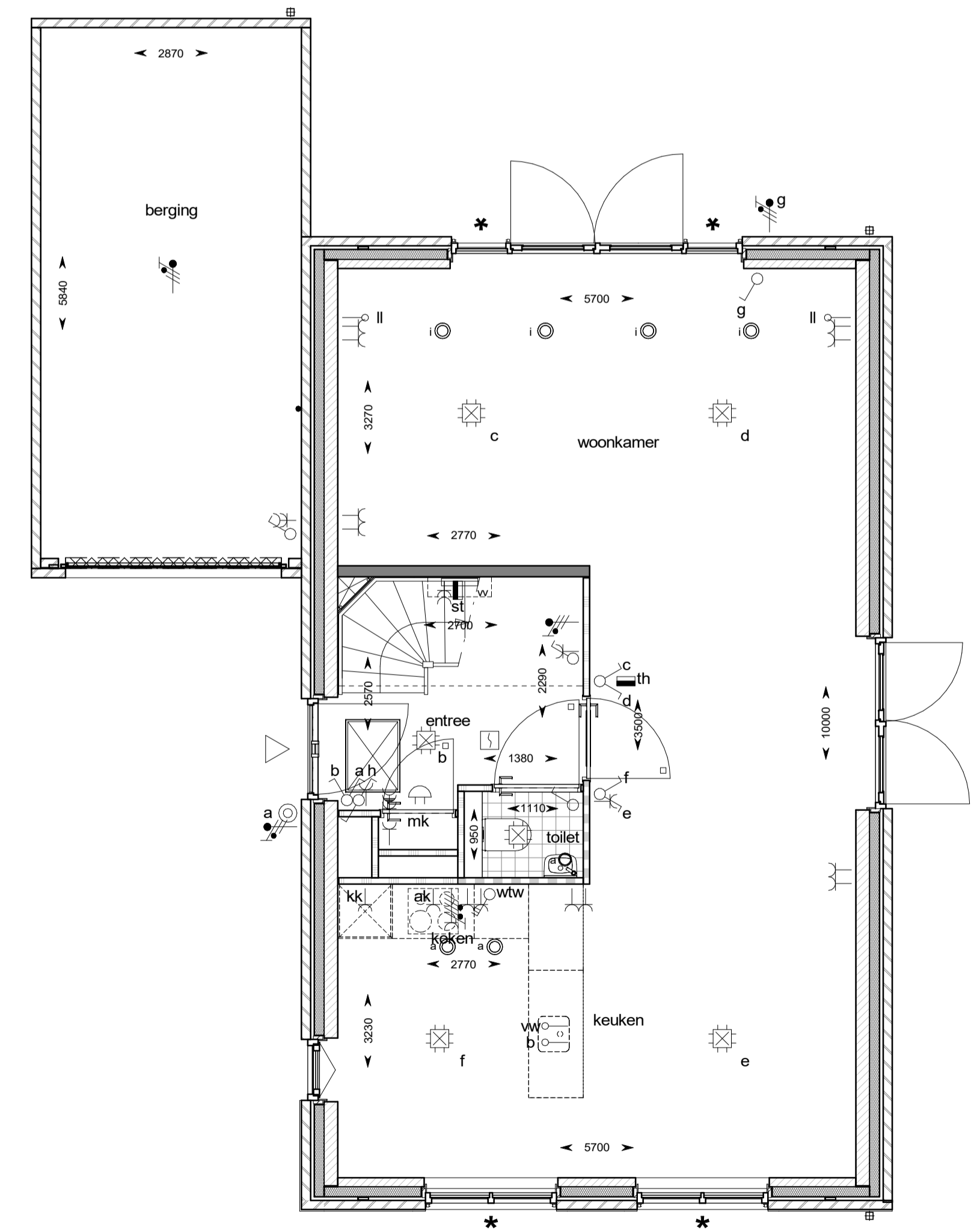
begane grond
