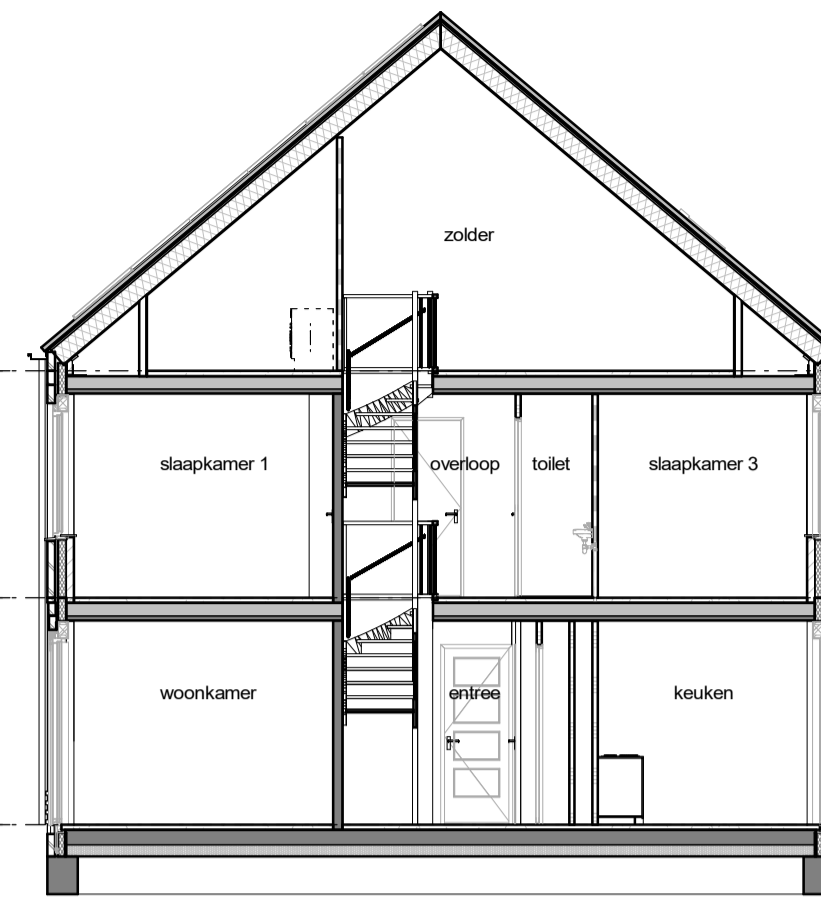
doorsnede
