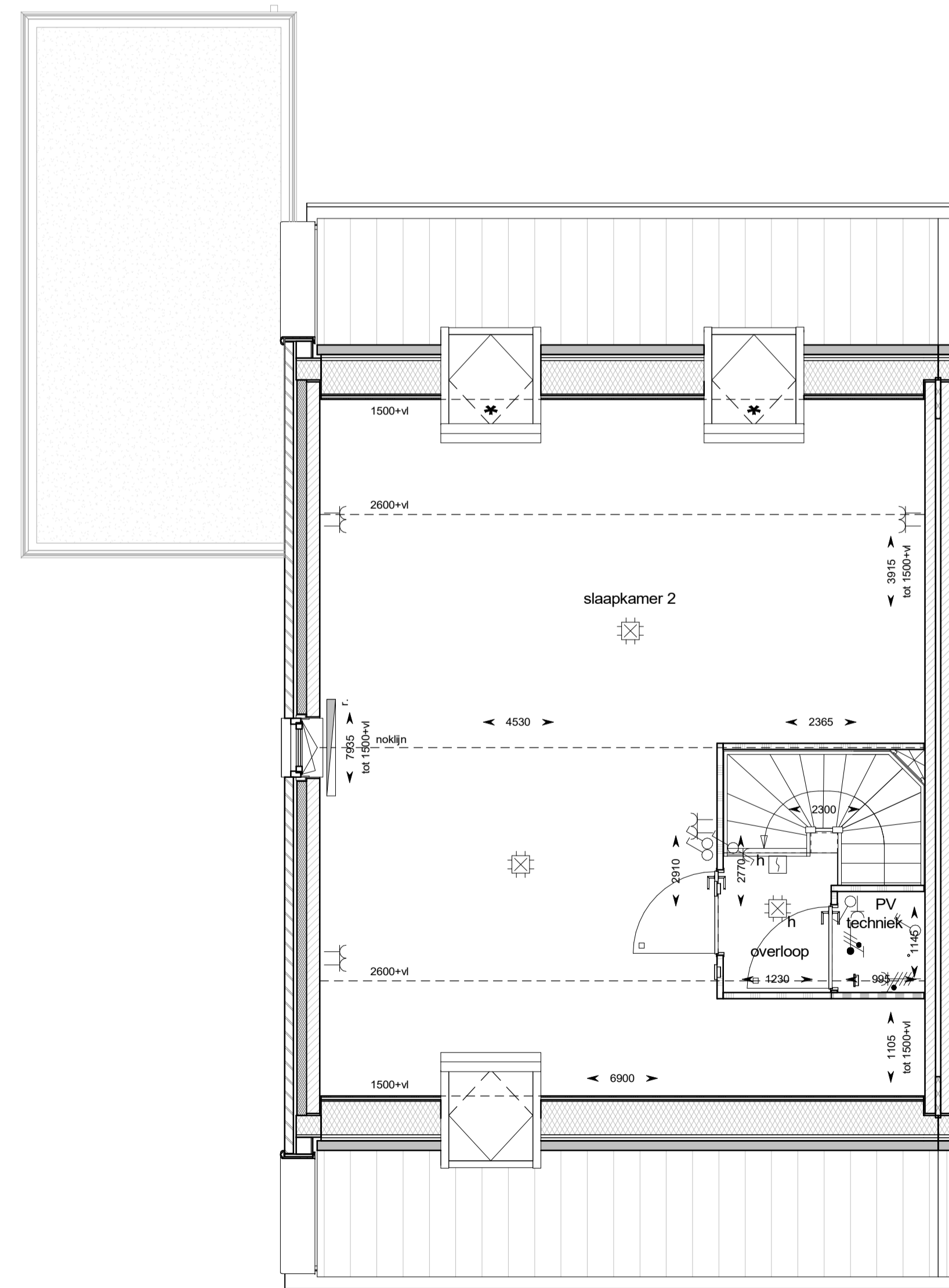
eerste verdieping
