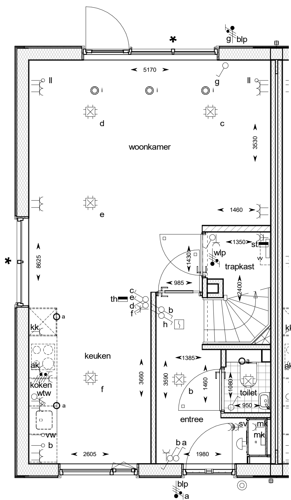
begane grond
