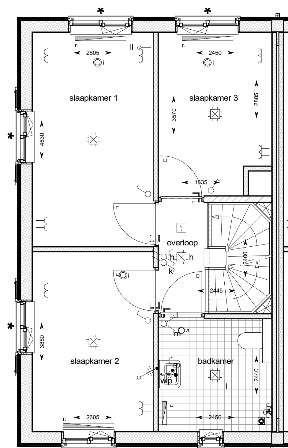
eerste verdieping
