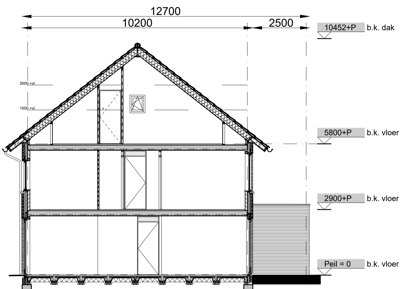
doorsnede A-A
