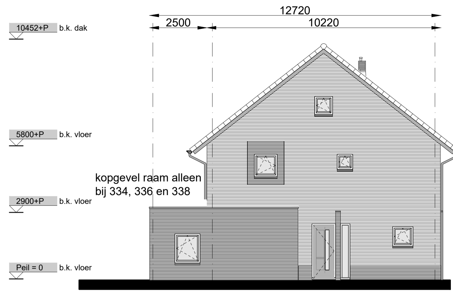
linker kopgevel
