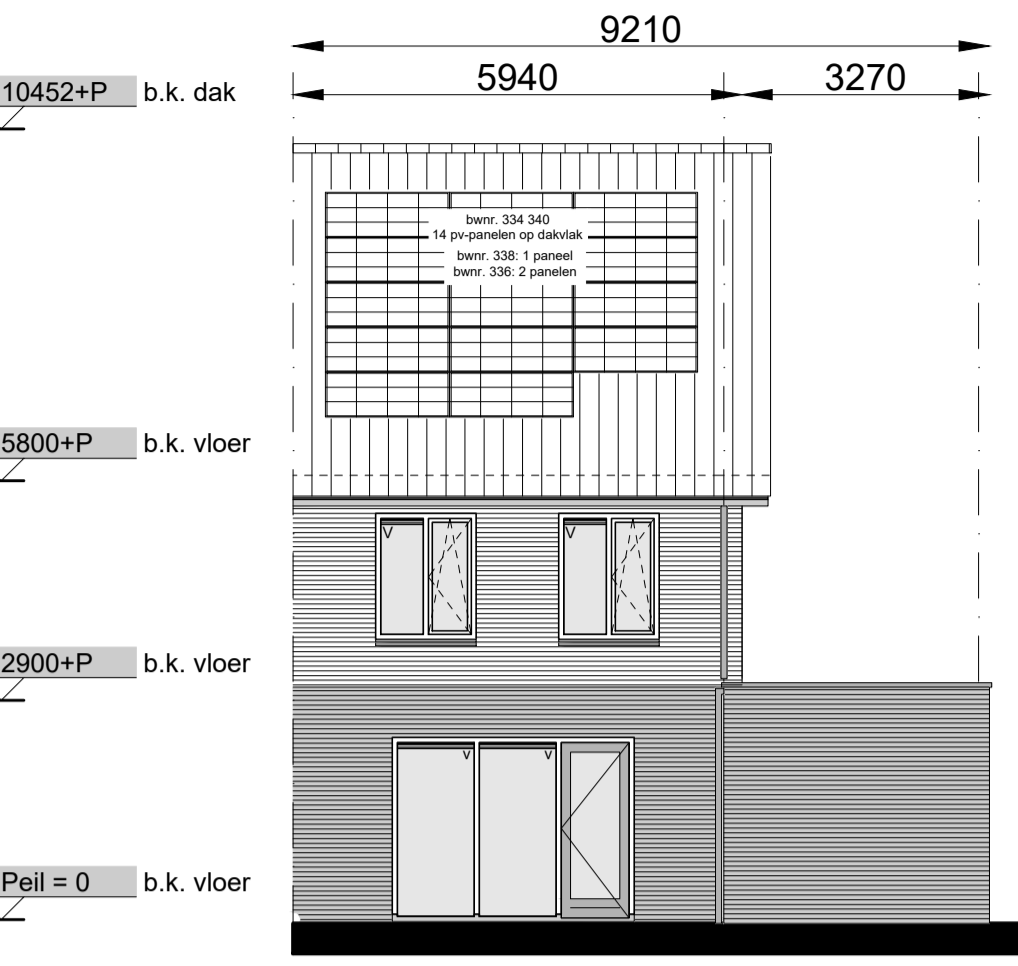
achtergevel
