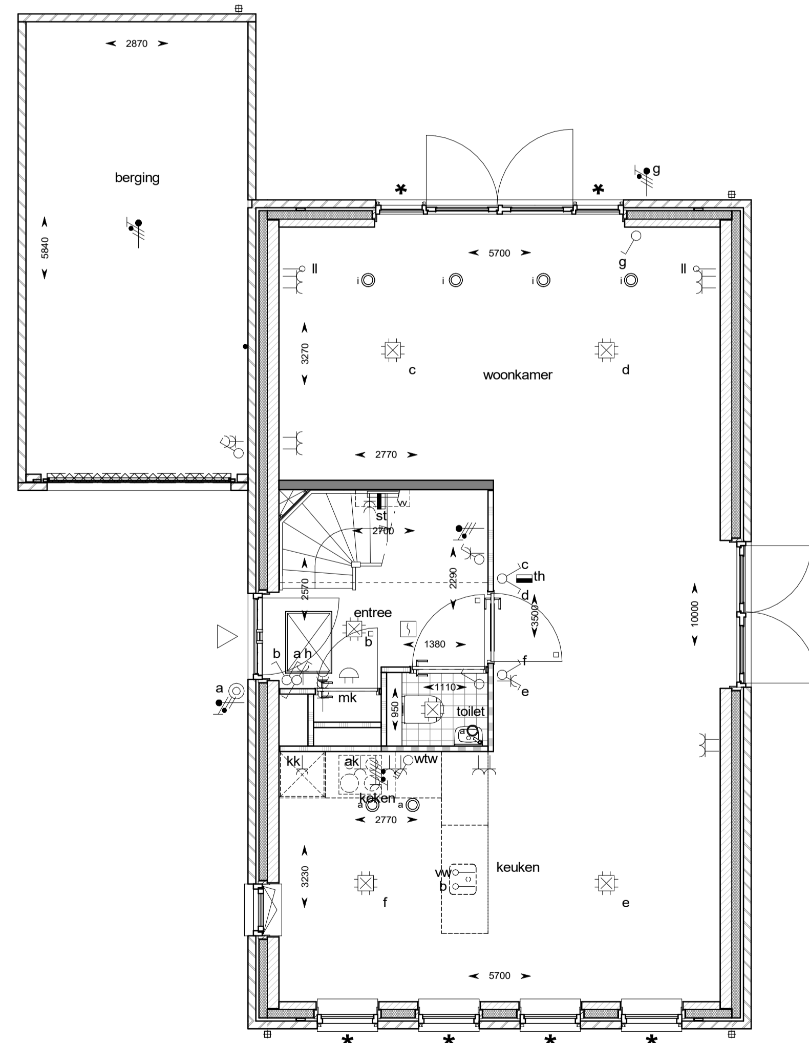
begane grond
