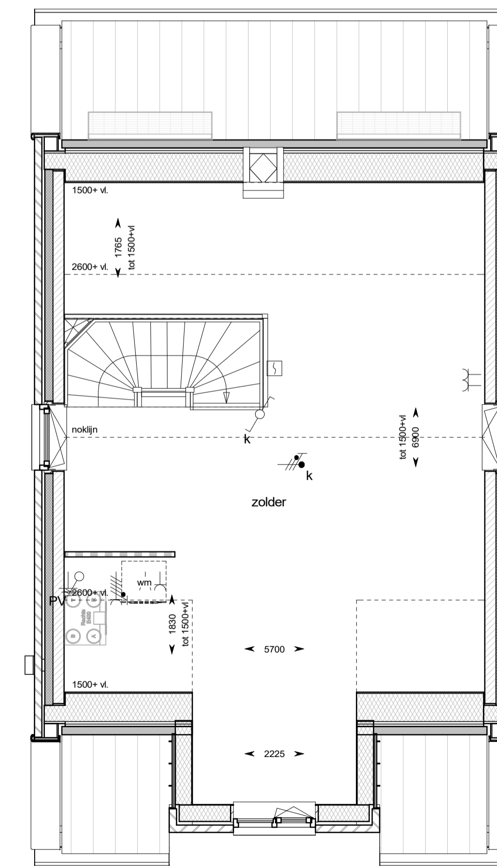
tweede verdieping
