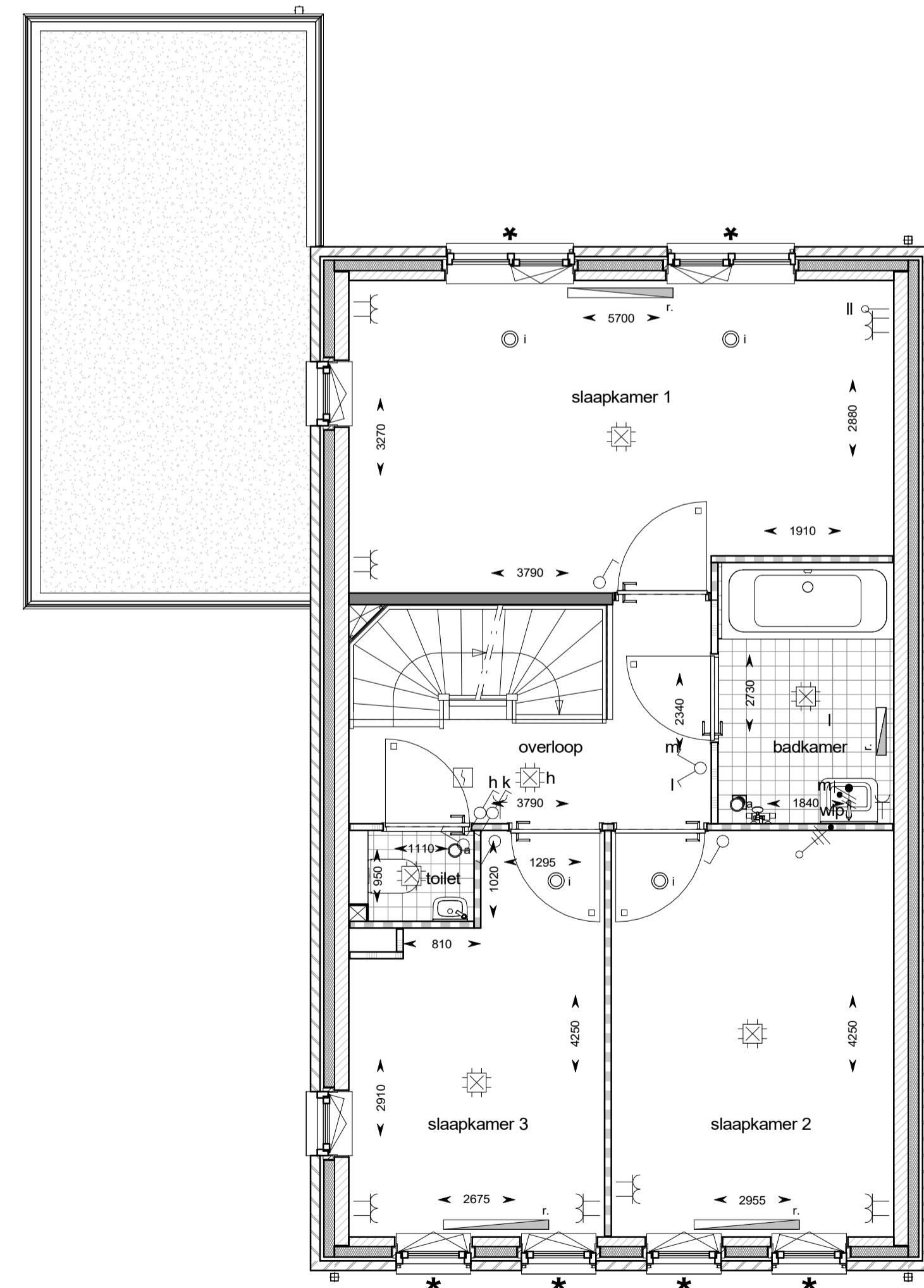
eerste verdieping
