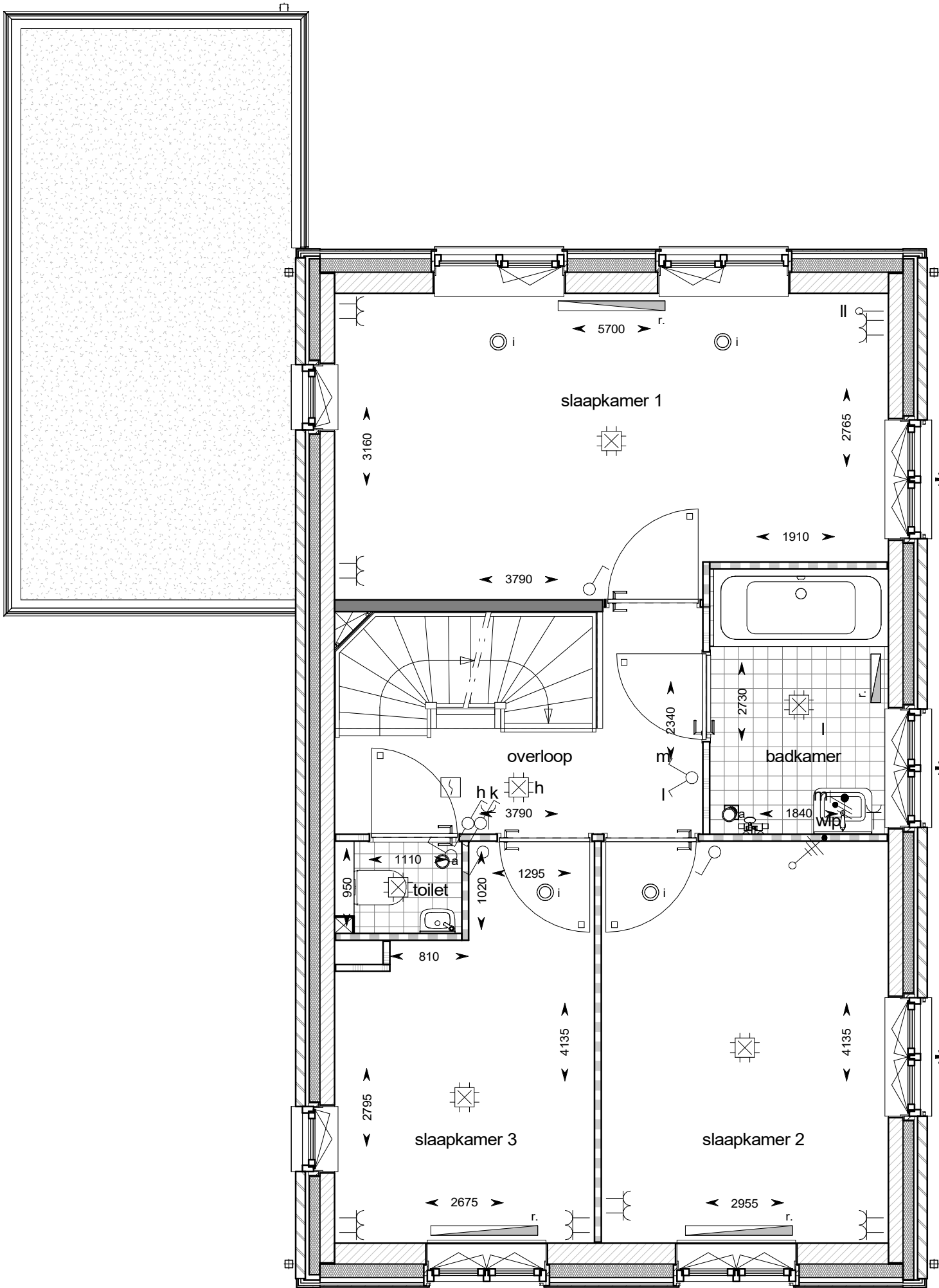
eerste verdieping
