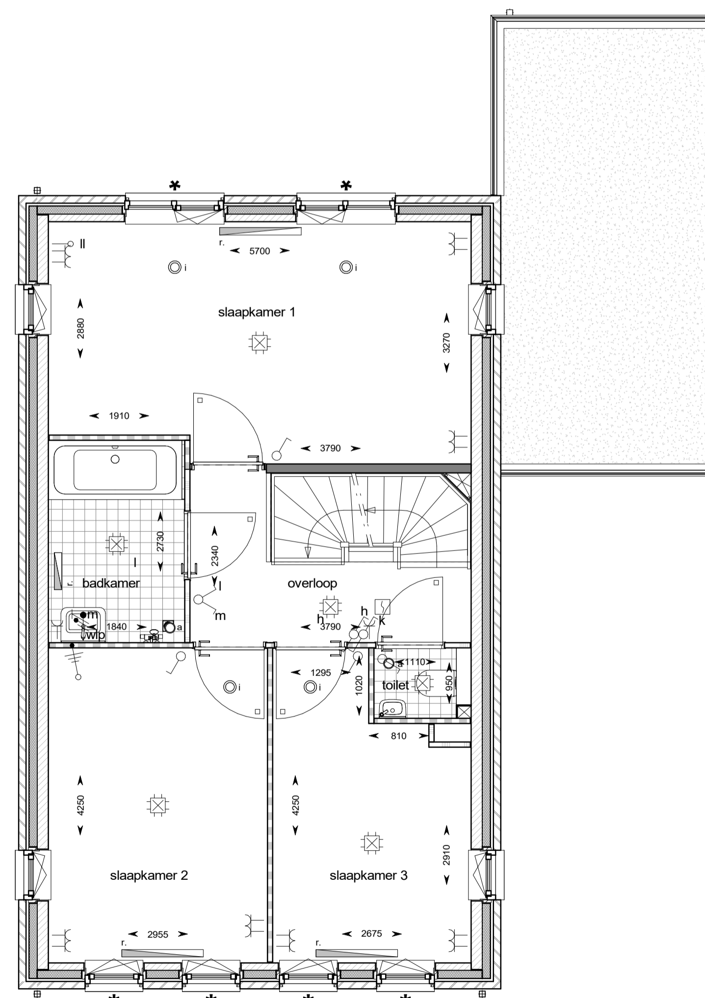
eerste verdieping
