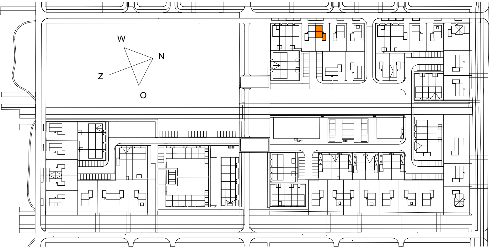
woningaanduiding 1 : 2000
