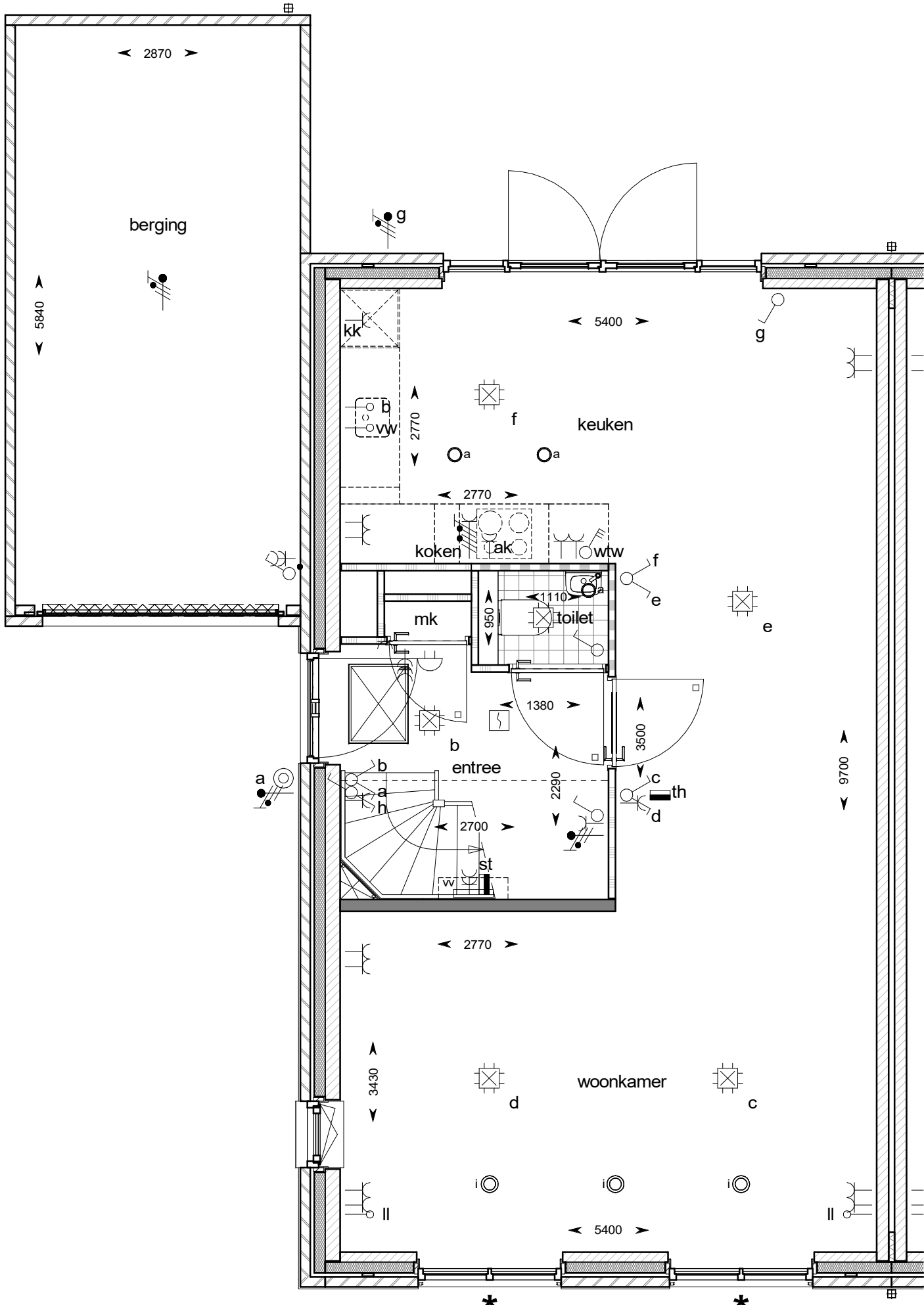
begane grond
