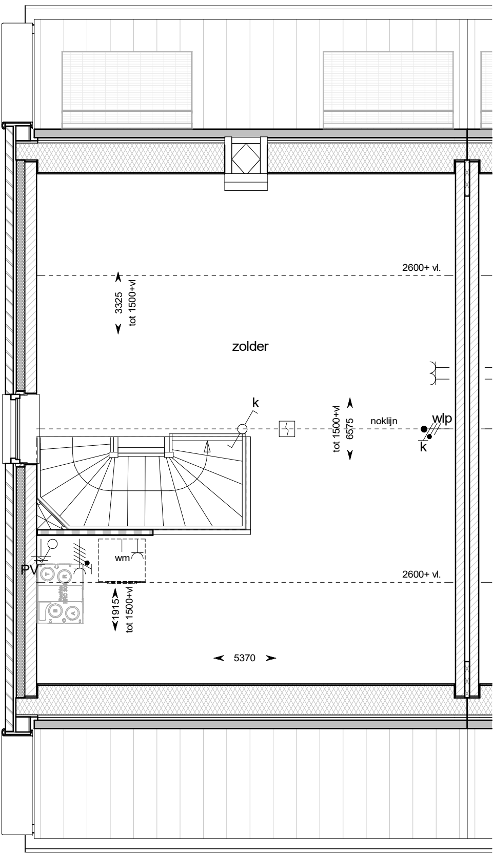
tweede verdieping
