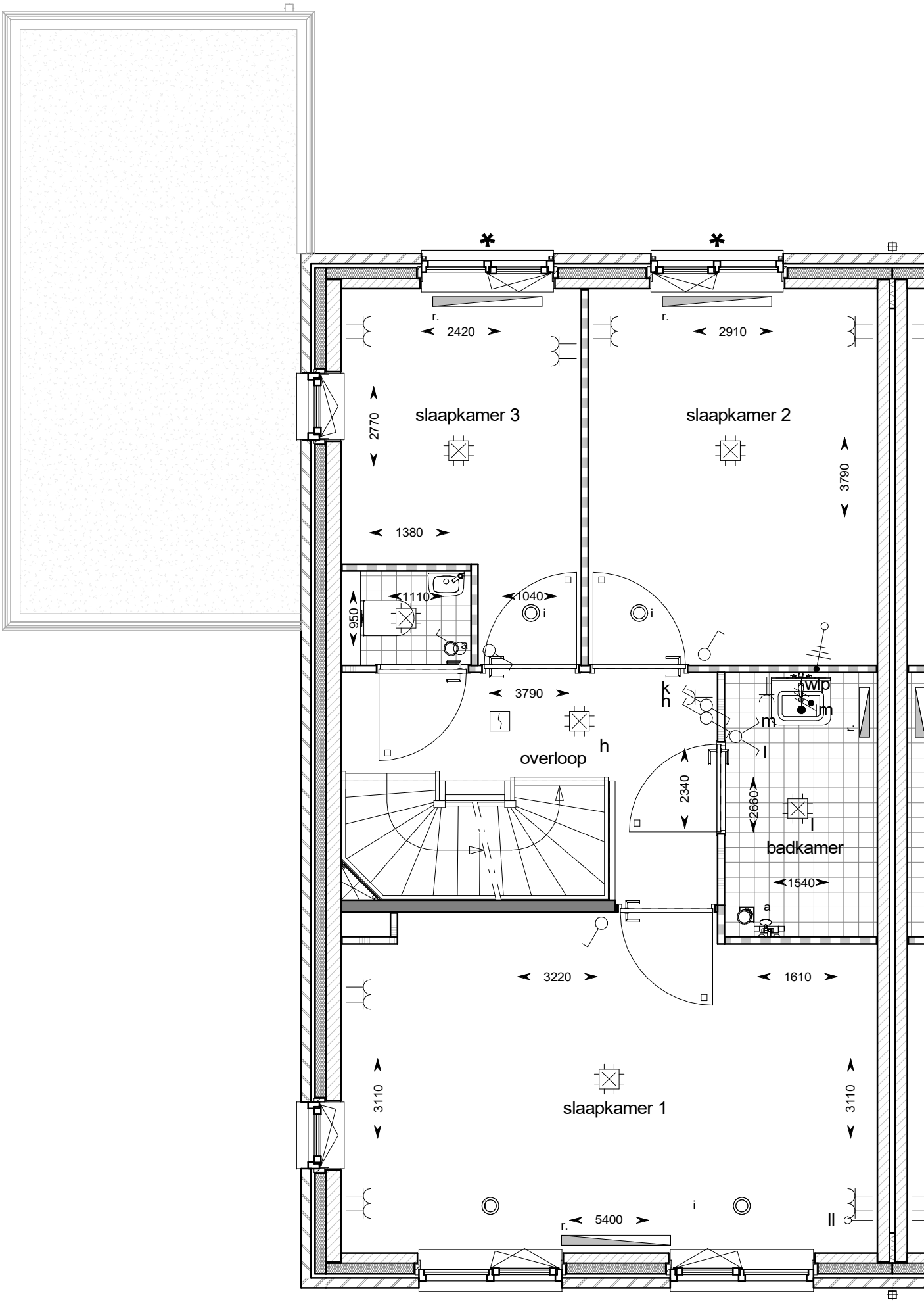
eerste verdieping
