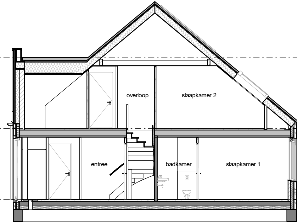
doorsnede
